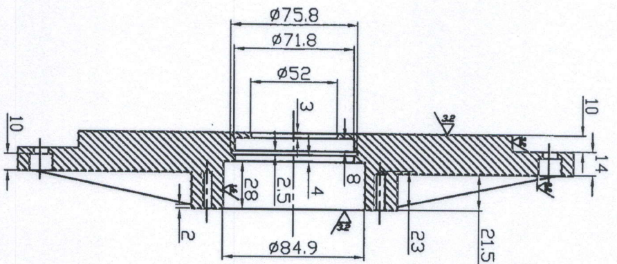
SEC A-A
