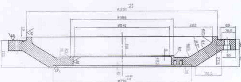
SEC A-A
