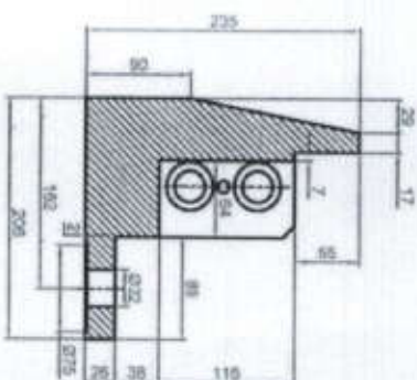
SFC A-A
